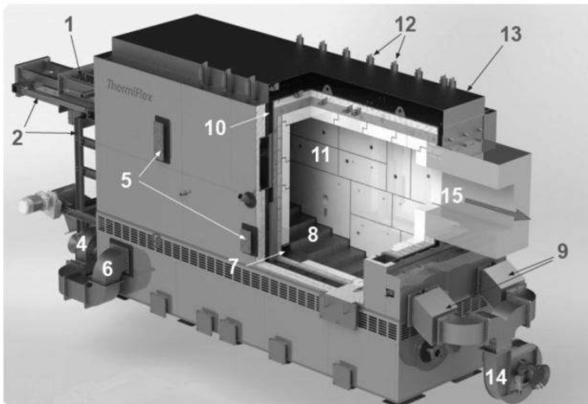
3. ábra: ThermiFlex hőerőmű felépítése 2.
