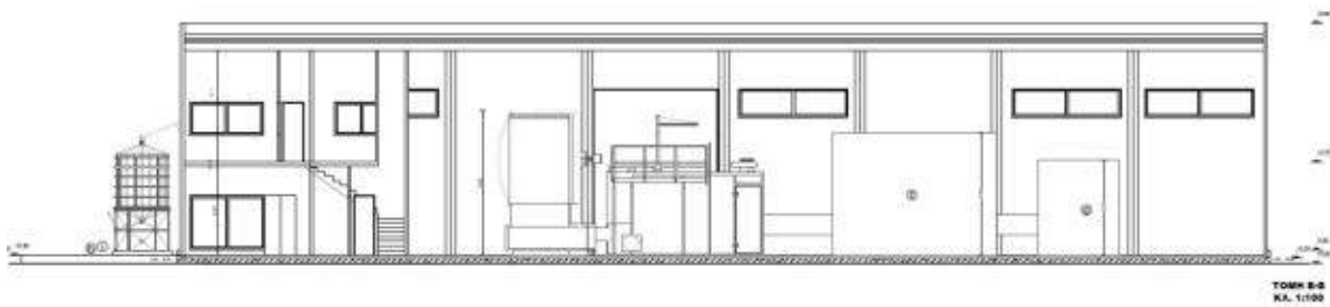
6. ábra: Tervezett építmény előzetes tervei 2.
